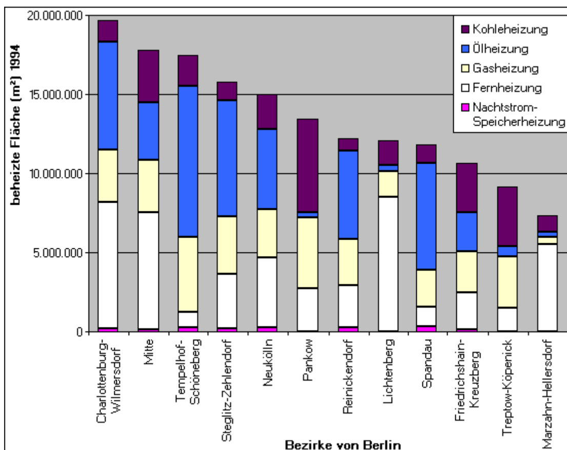
Abb. 1: Wohn- und Gewerberaumheizung pro Bezirk 1994
