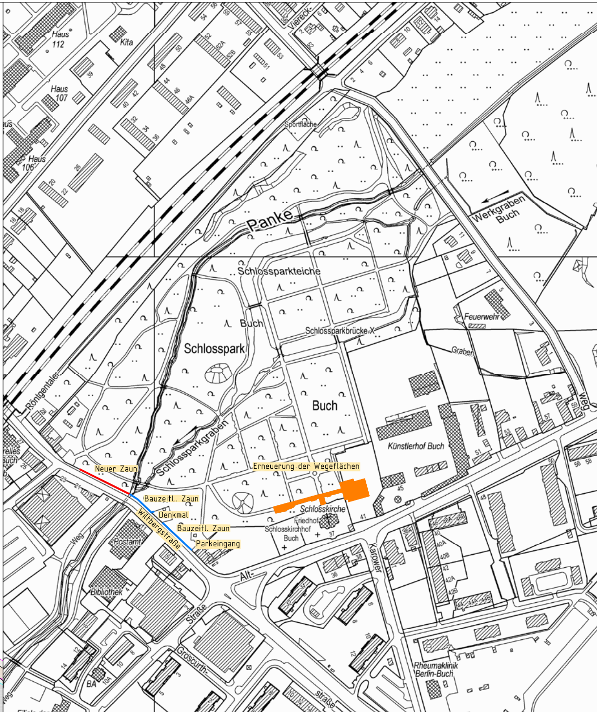
Lageplan ohne Maßstab
