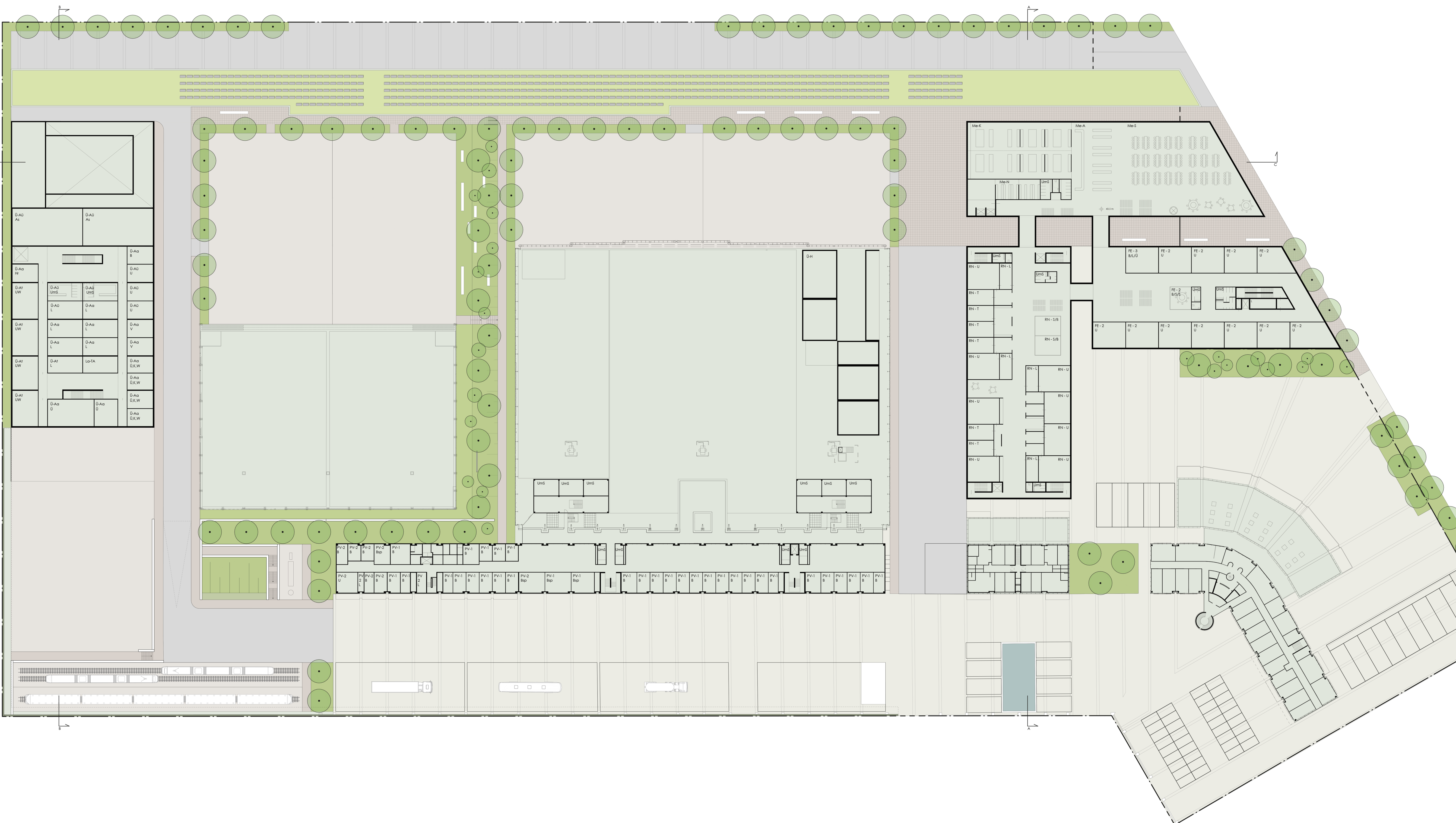
Grundriss 1. Obergeschoss
