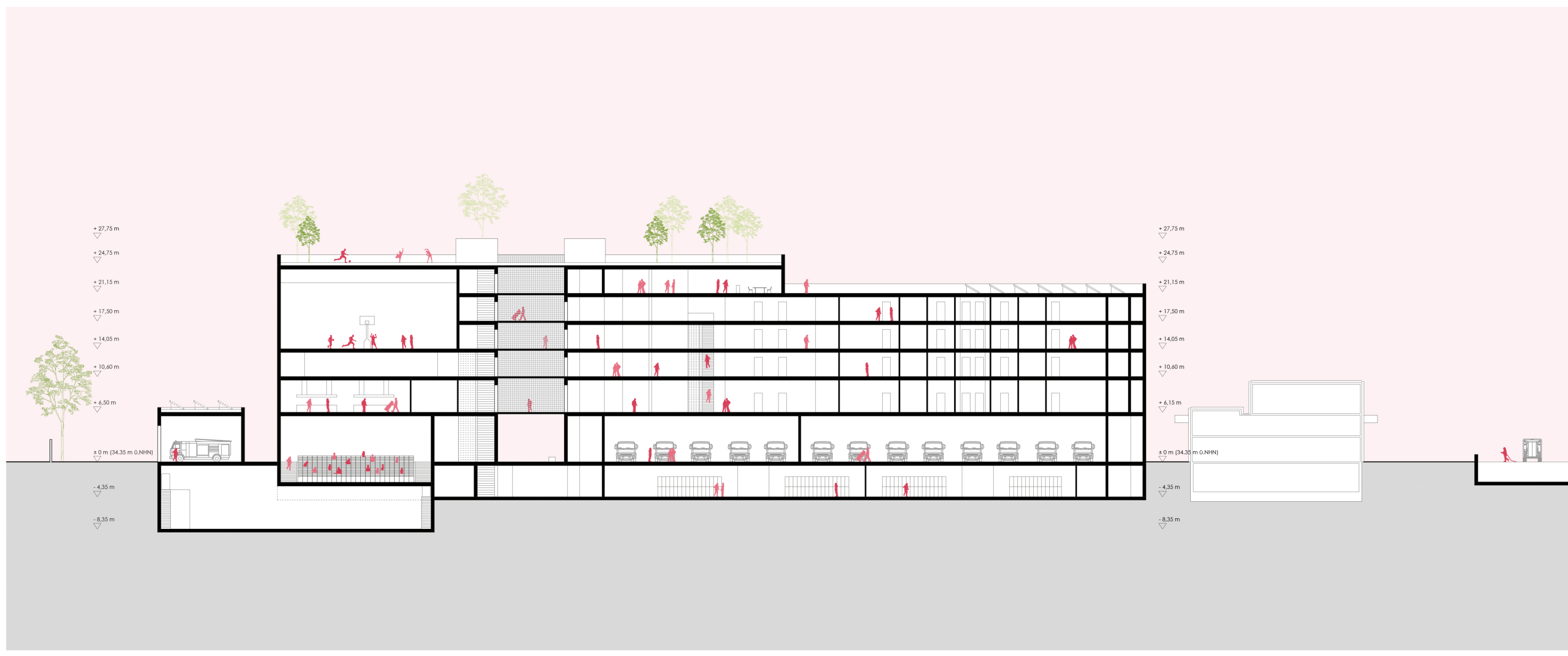
Schnitt AA
