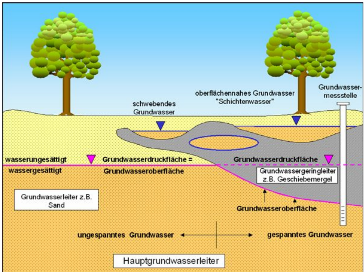
Abb. 3: Hydrogeologische Begriffe
