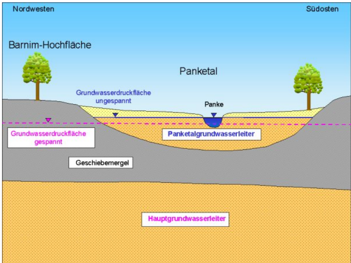
Abb. 8 Der ungespannte Panketalgrundwasserleiter (GWL 1) im nordwestlichen Bereich der Barnim-Hochfläche liegt über dem Hauptgrundwasserleiter (GWL 2), der hier gespannt ausgebildet ist
