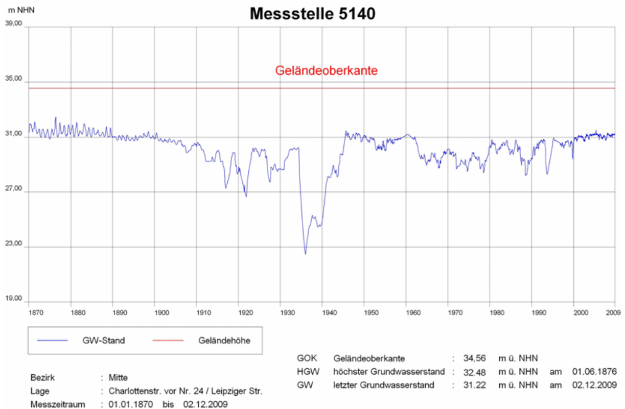
Abb. 9: Grundwasserstandsganglinie einer Messstelle aus der Innenstadt von 1870 bis heute. Der höchste Grundwasserstand (HGW) wurde hier am 1.6.1876 gemessen. Der Grundwasserstand ist durch zahlreiche Grundwasserabsenkungen seit 1905 zeitweise stark beeinflusst.
