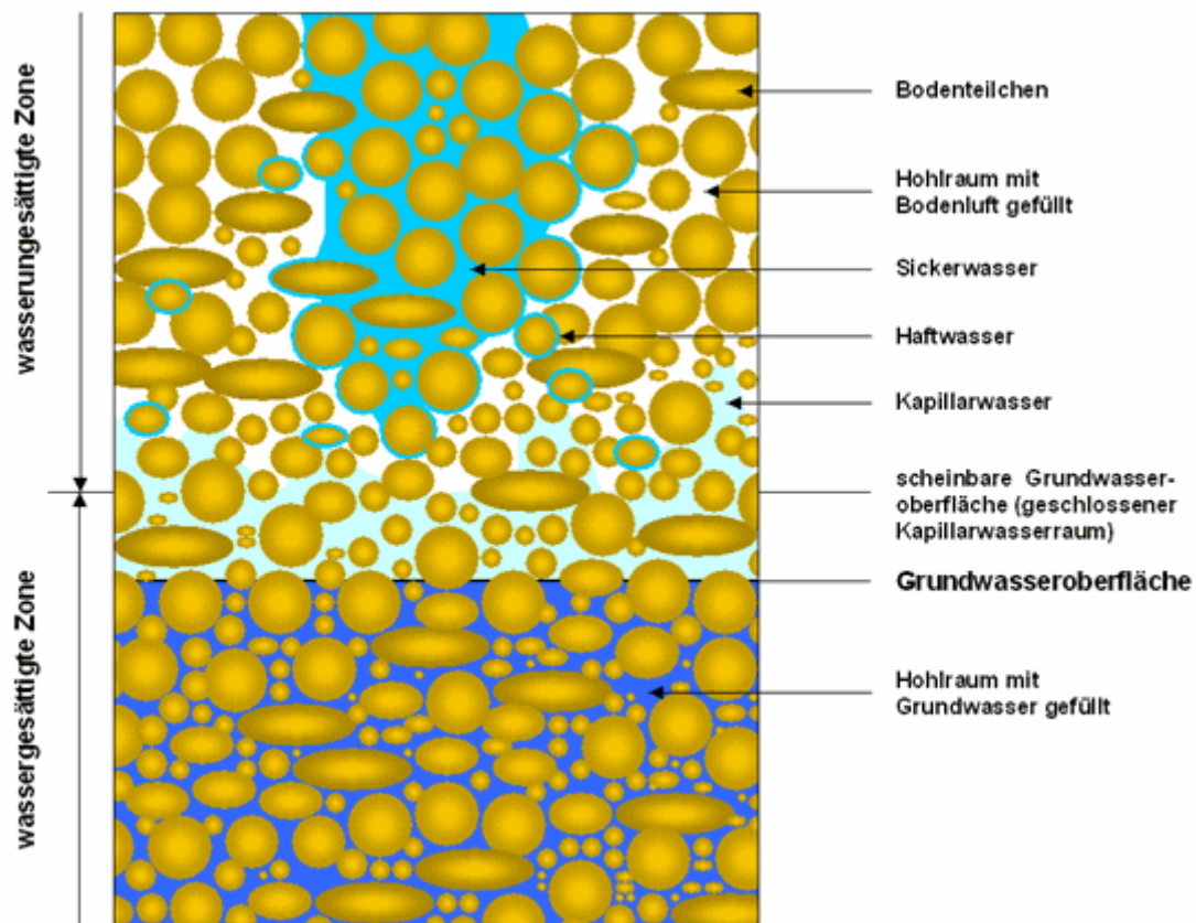
Abb. 2: Erscheinungsform des unterirdischen Wassers (aus Hölting 1996)
