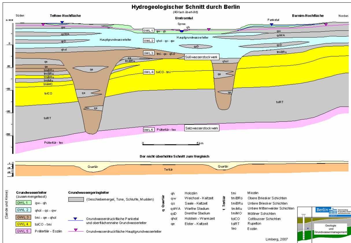
Abb. 7: Schematischer Hydrogeologischer Schnitt von Süden nach Norden durch Berlin
