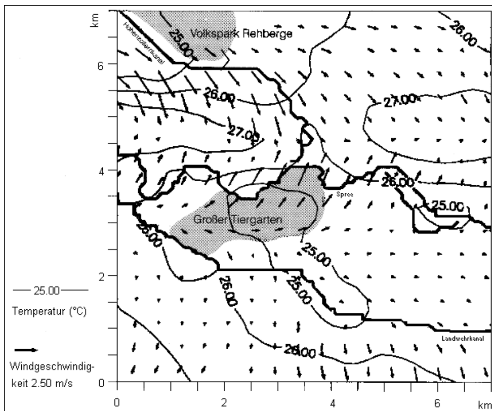
Abb. 1: Simulation des Temperatur- und Windfeldes in 10 m Höhe im Innenstadtbereich von Berlin während einer sommerlichen Strahlungswetterlage um 14.00 Uhr MEZ unter Berücksichtigung der Flächennutzung im Jahre 1993. Initialisierung des Modells mit Wind aus West mit 3m/s (aus: Wagner 1993, leicht verändert).
