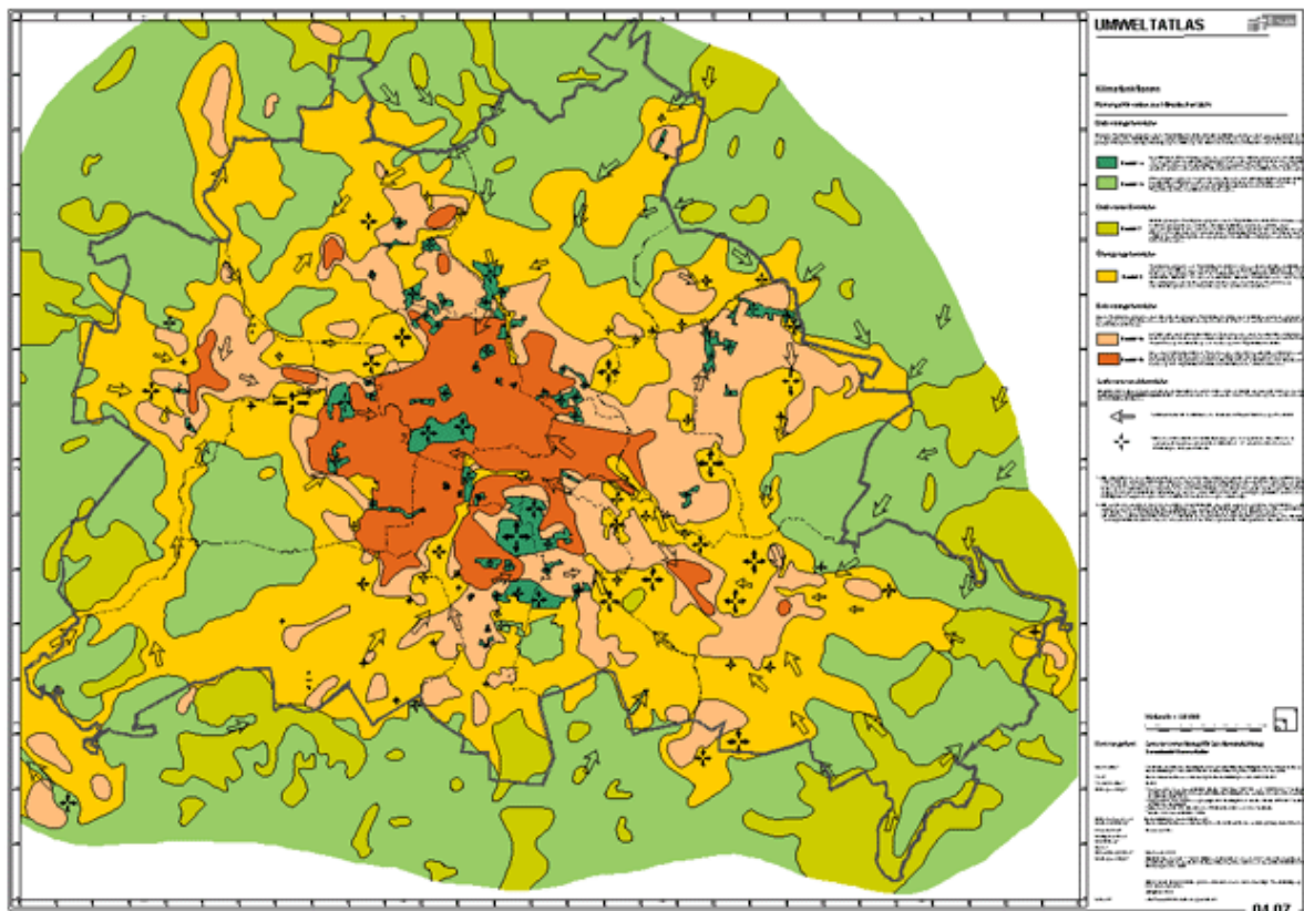
Abb. 3: Ehemalige Klimafunktionskarte (04.07) des Umweltatlas Berlin (Stand 2001)
