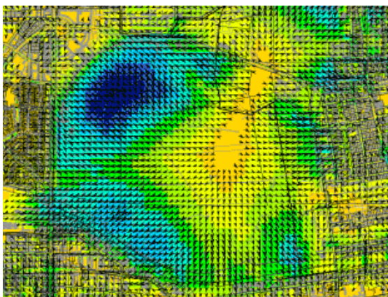
Abb. 2: Bodennahe Strömungsfeld und Kaltlufteinwirkbereich des Flughafens Tempelhof
