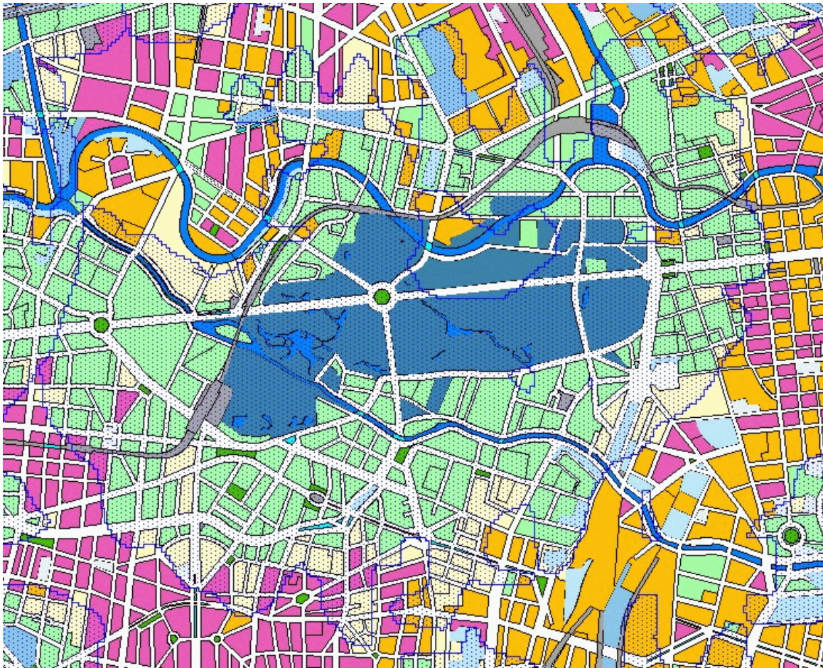
Abb. 5: Simulierter Einwirkbereich der im Großen Tiergarten produzierten Kaltluft
