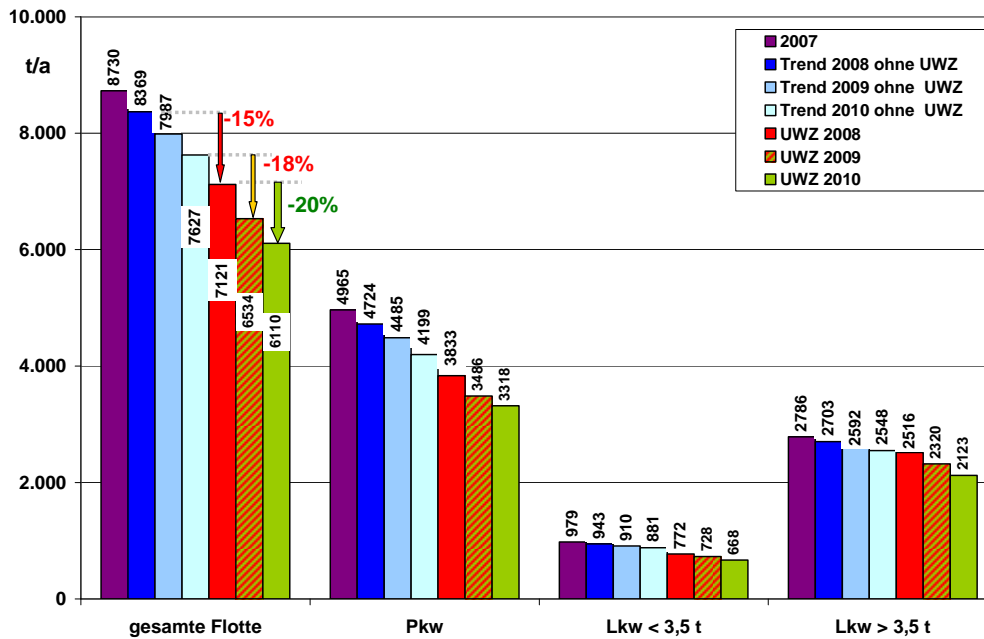
Abbildung 3.7: Veränderung der Emissionen von Stickoxiden (ohne Kaltstartbeiträge) in Berlin nach HBEFa 3.1 aufgrund der Umweltzone (Flottenzusammensetzung an der Frankfurter Allee; gleiche Verkehrsleistungen; ohne Kaltstartemissionen)
